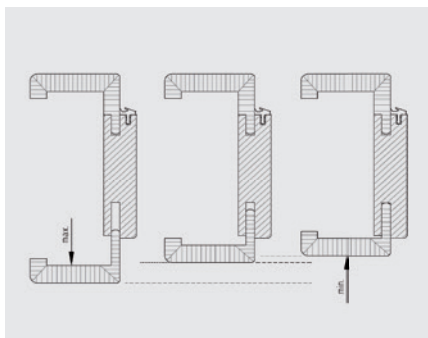
Aanpasbaarheid wanddikte (stelbereik - 5 mm, + 15 mm).
