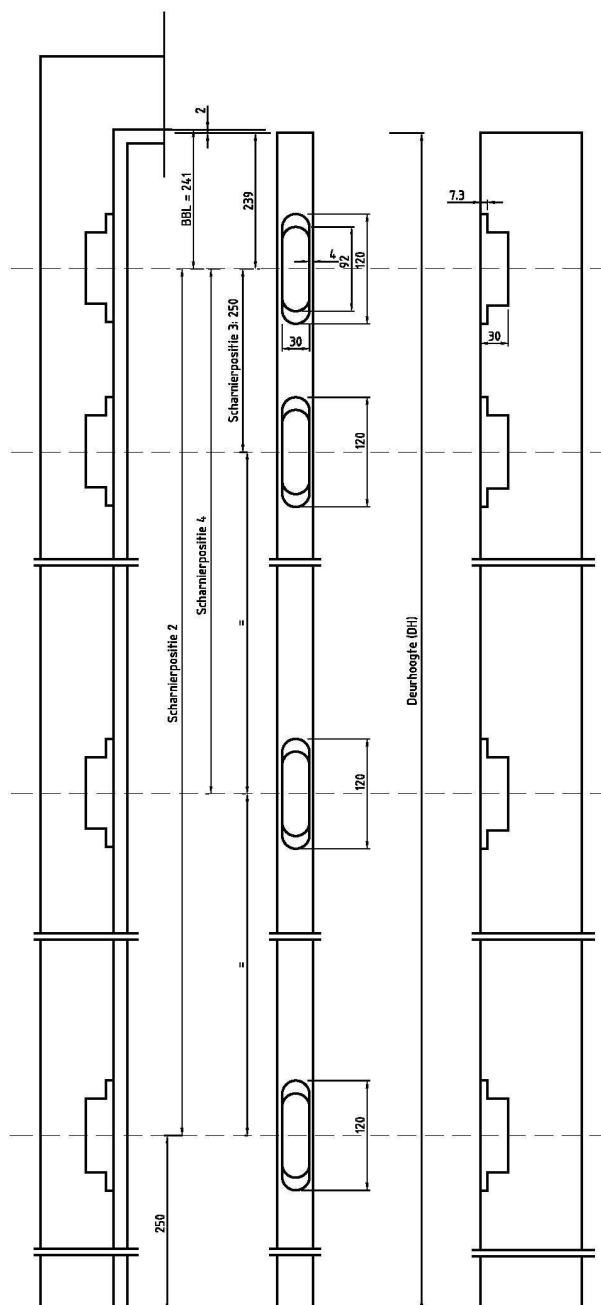
3 of 4 scharnieren
