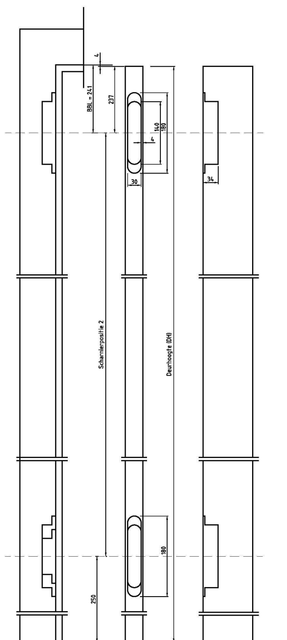
2 scharnieren
