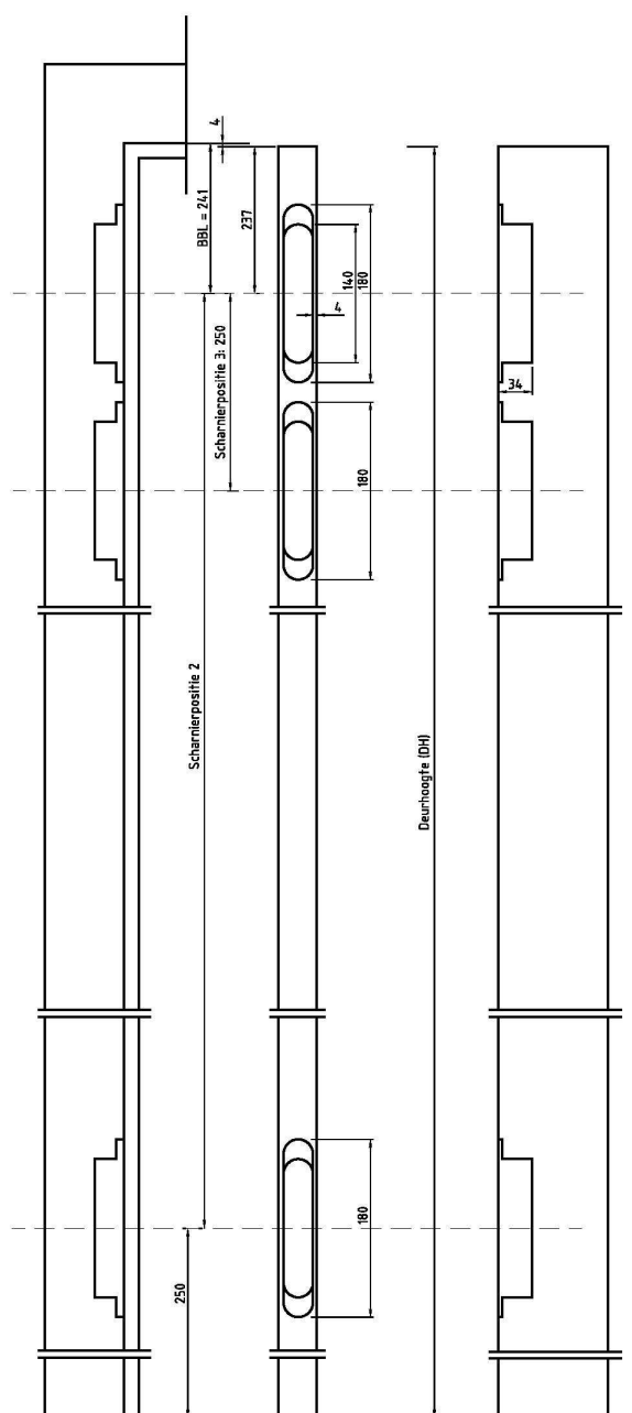
3 scharnieren
